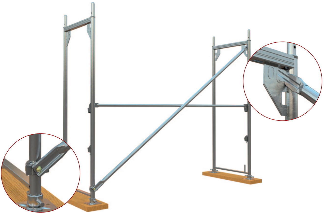
Rys. 4. Montaż stężenia ukośnego pierwszego pola
